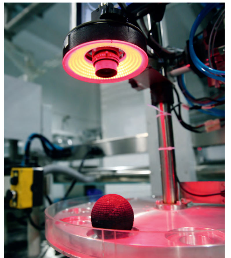
高温气冷堆球形燃料元件
